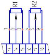
Рисунок В3 – схема с БСПИ-10 остальное – см. рисунок В.1 или В.2
