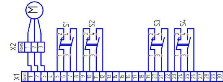
Рисунок В3 – схема с БСПИ-10 остальное – см. рисунок В.1 или В.2
