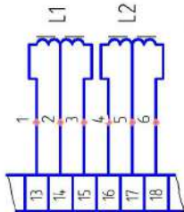
Рисунок В3 – схема с БСПИ-10 остальное – см. рисунок В.1 или В.2
